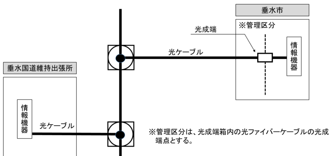
別図 1 光ファイバーケーブル等の施工及び管理区分の責任分解
